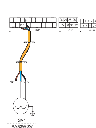
Rys. 3. Schemat podłączenia zaworu do pompy ciepła Rotenso Aquami
