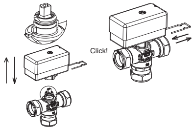
Rys. 8. Montaż siłownika
