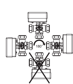
Rys. 9. Pozycje montażowe
