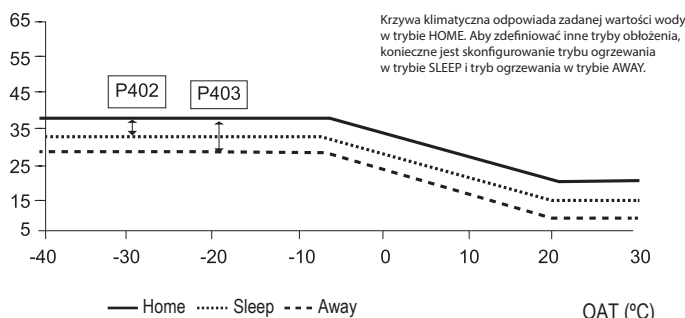
Krzywe klimatyczne w trybie grzania w zależności od wybranego trybu użytkowania
