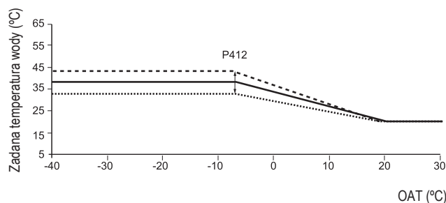
Ogrzewanie chłodzenie krzywa klimatyczna: przesunięcie na czele krzywej
