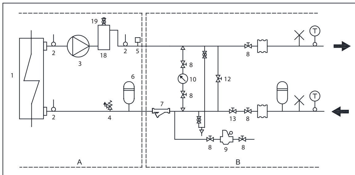
Rysunek 7: Przykładowy schemat obwodu hydraulicznego dla jednostek 12-16 kW
