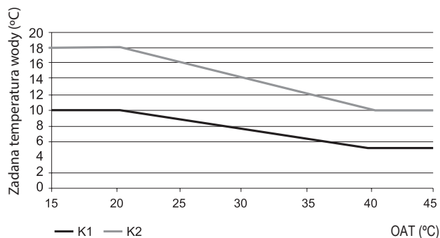
Krzywe klimatyczne w trybie chłodzenia
