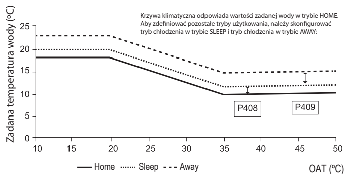
Krzywe klimatyczne w trybie chłodzenia w zależności od wybranego trybu użytkowania
