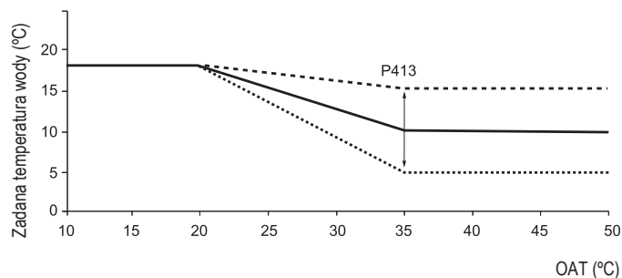
Niestandardowa krzywa klimatyczna chłodzenia: przesunięcie na stopie krzywej
