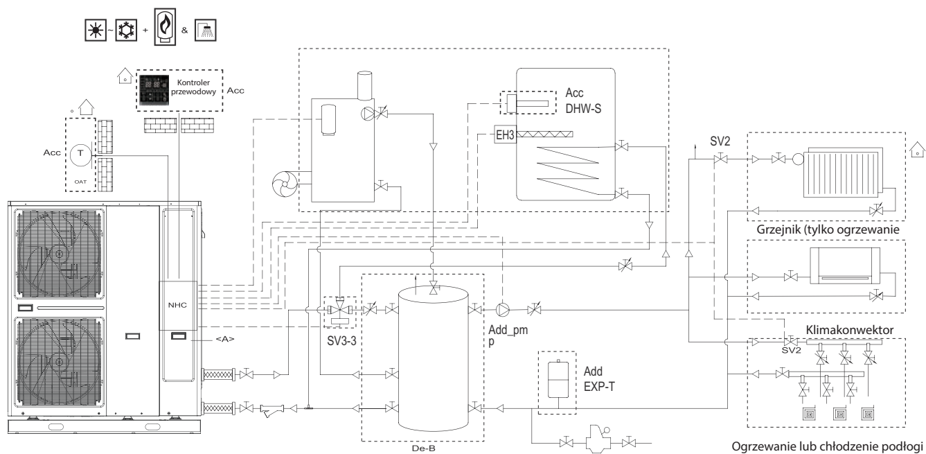
Rysunek 10: Standardowa instalacja ze zbiornikiem CWU i dodatkowym źródłem grzewczym (AHS)
