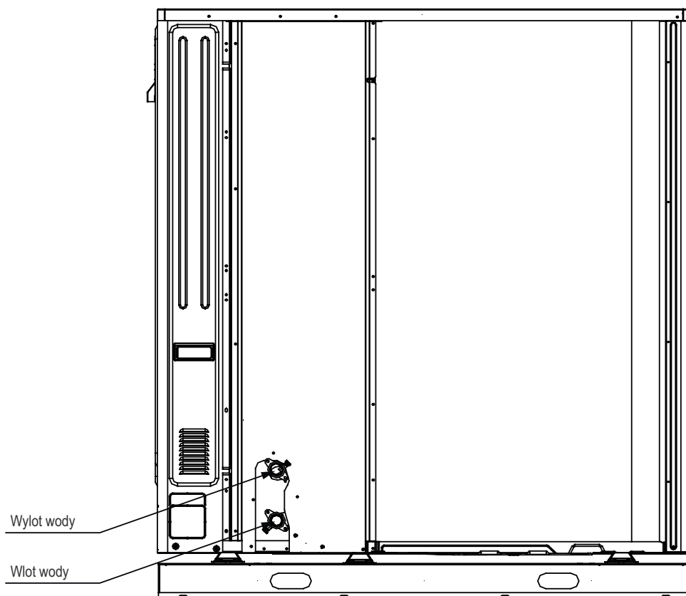
Rysunek 5: Przyłącza wodne w urządzeniu
