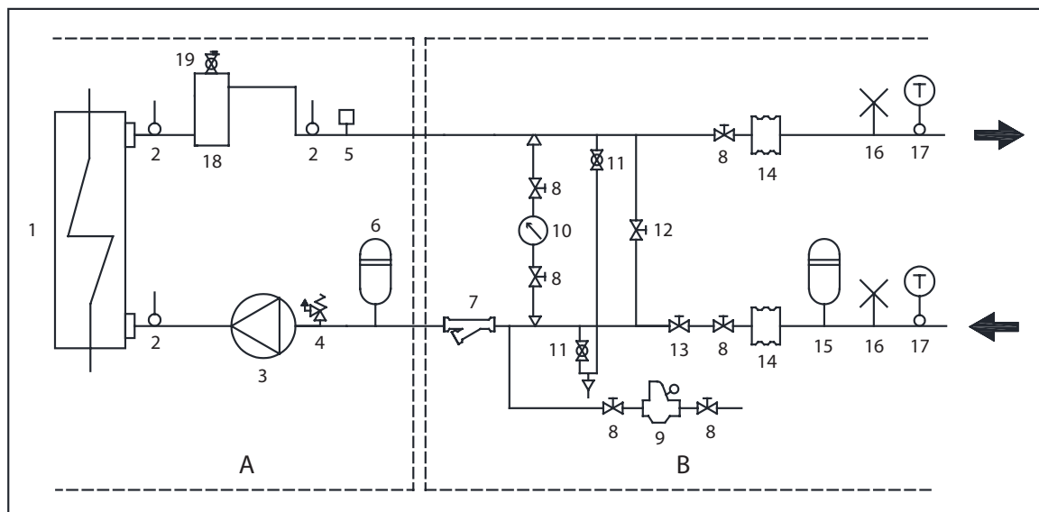
Rysunek 6: Przykładowy schemat obwodu hydraulicznego dla jednostek 4-10 kW
