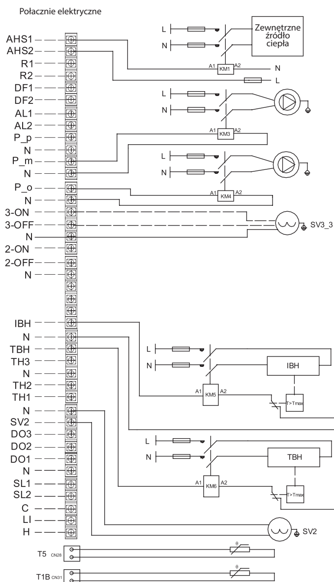
Rysunek 10: Standardowa instalacja ze zbiornikiem CWU i dodatkowym źródłem grzewczym (AHS)
