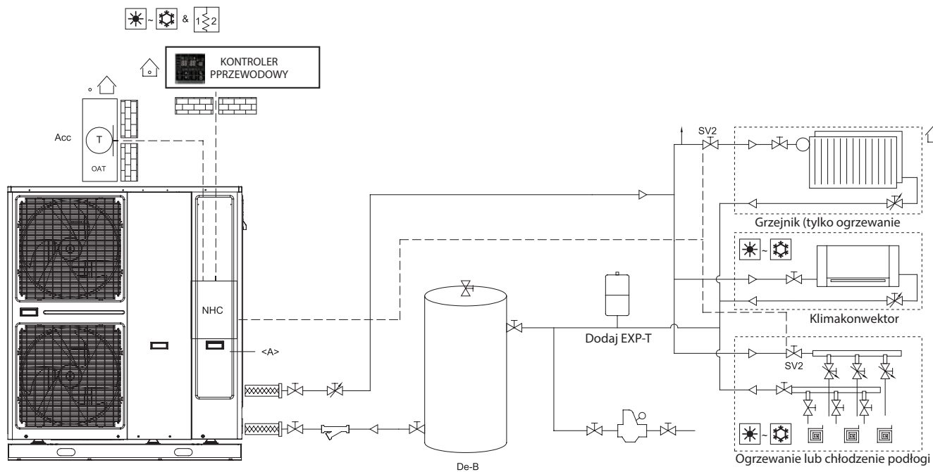
Rysunek 10: Standardowa instalacja z elektryczną grzałką wspomagającą
