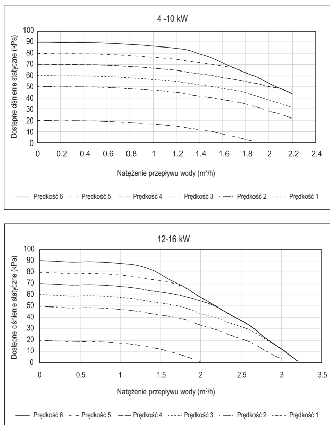
Grafika 1: Dostępne ciśnienie statyczne dla jednostek 4 do 16 kW
