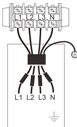
ZASILANIE JEDNOSTKI WEWNĘTRZNEJ (3 fazowe)
