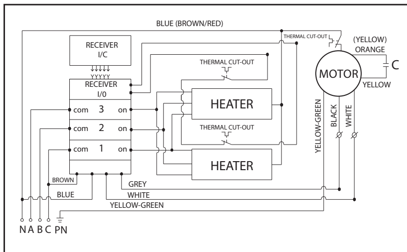
3 fazy (400V~), główna linia: A, B, C, N
