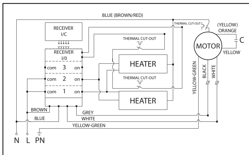
1 faza (230V~), główna linia: L, N
